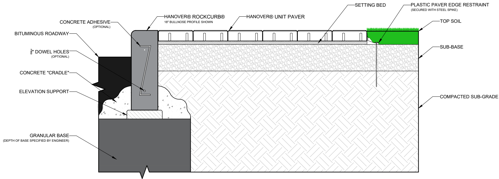
LONGITUDINAL SECTION
